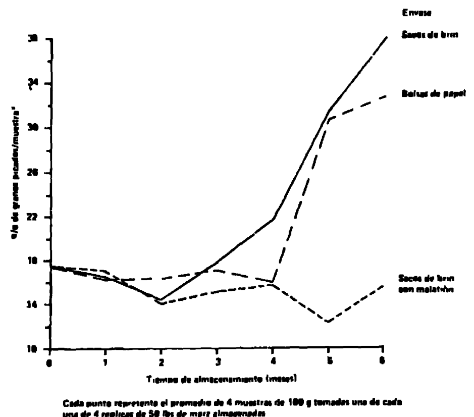
Fig 1 Proceso de deterioro del maíz Opaco-2 almacenado durante 6 meses en 3 tipos de envase
