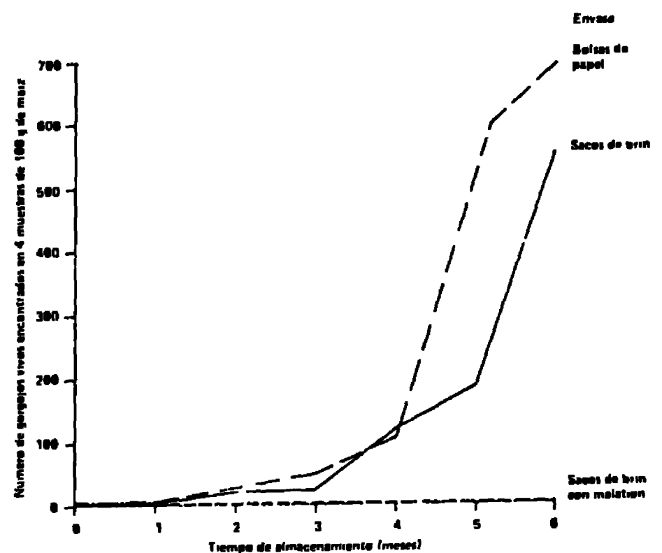
Fig 2 Proceso de infestación por gorgojos ( Sitophilus sp.) del maíz Opaco 2 almacenado durante 6 meses en 3 tipos de envase
