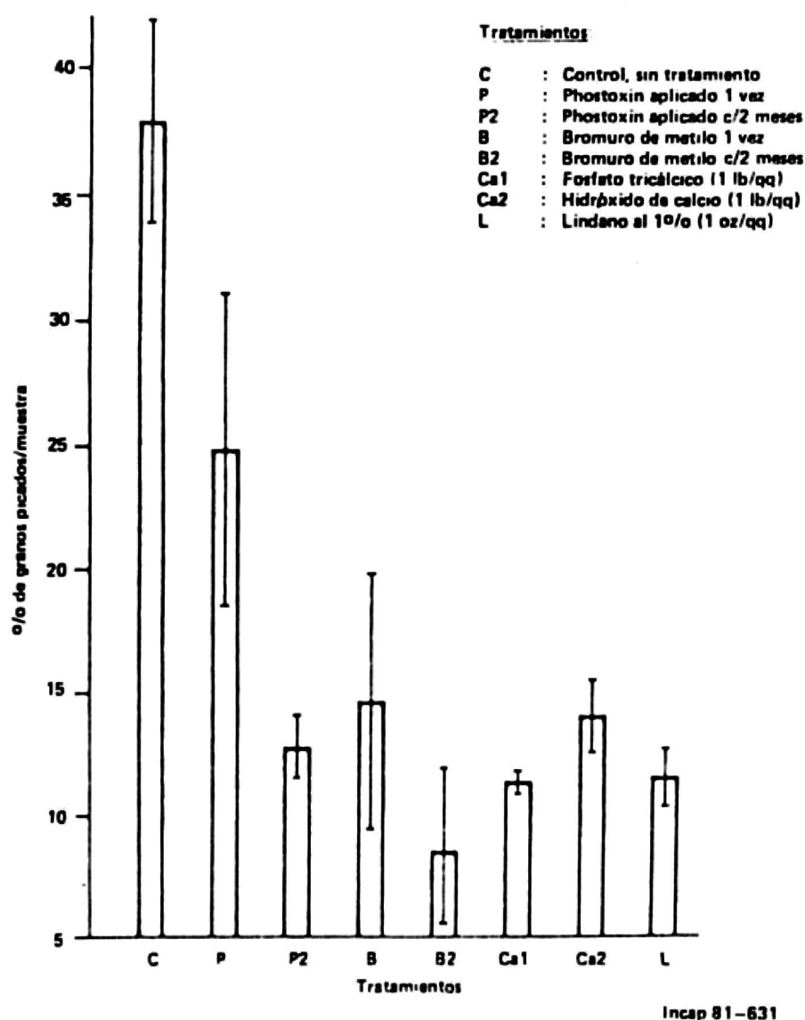
Fig. 3. Daño ocasionado por insectos al grano del maíz Opaco-2 después de 6 meses de almacenamiento en sacos de brin, aplicándose diferentes tratamientos. (Promedio \pm F. E., n = 4 ).
